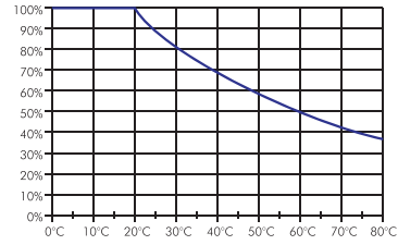
Druck/Temperaturdiagramm PUN-Schläuche
